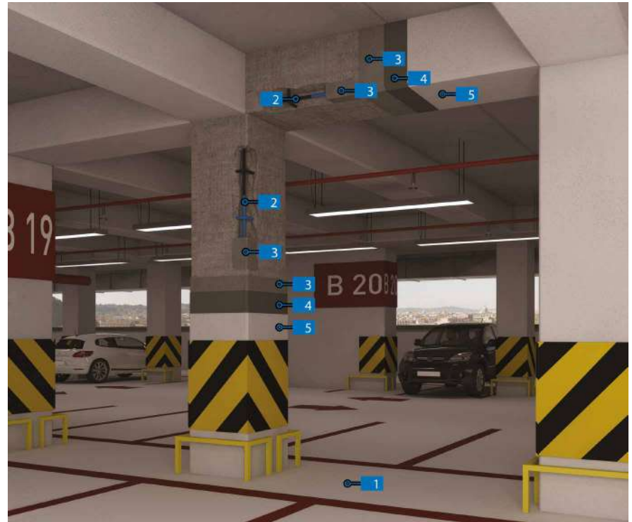
REHABILITACIÓ DE PARKING COMUNITARIS AMB SISTEMA DURADOR PER A LA PROTECCIÓ I REPARACIÓ ESTRUCTURAL D'ELEMENTS DE FORMIGÓ ARMAT AMB ACABAT ELASTOMÈRIC
